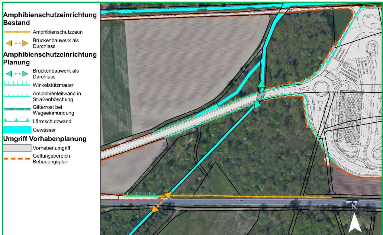
Abb. 20. Amphibienschutzeinrichtungen, unmaßstäblich
